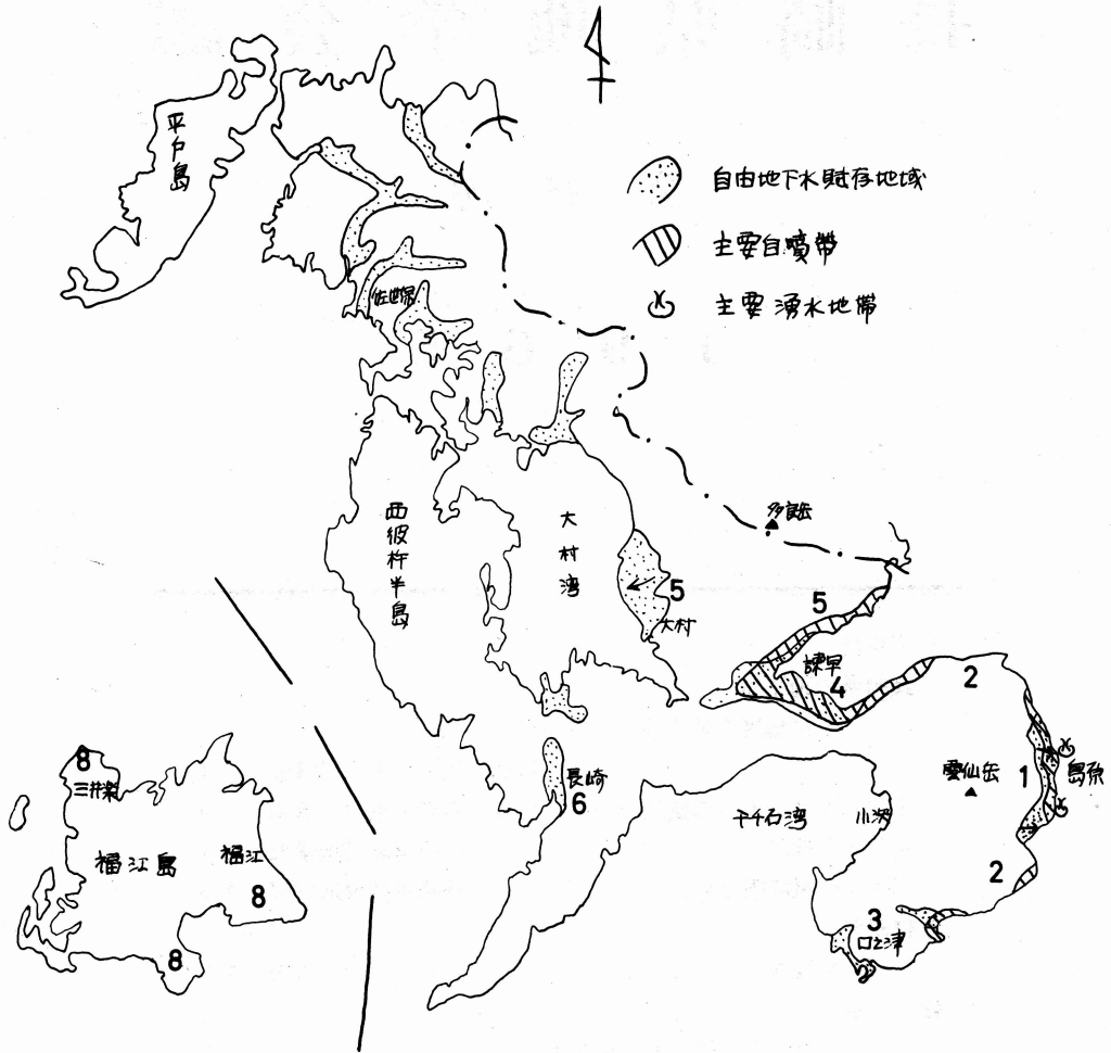
長崎県における地下水分布概略図 (古川博恭原図)
